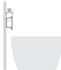
Estante a pared para grifería de 120x20h
